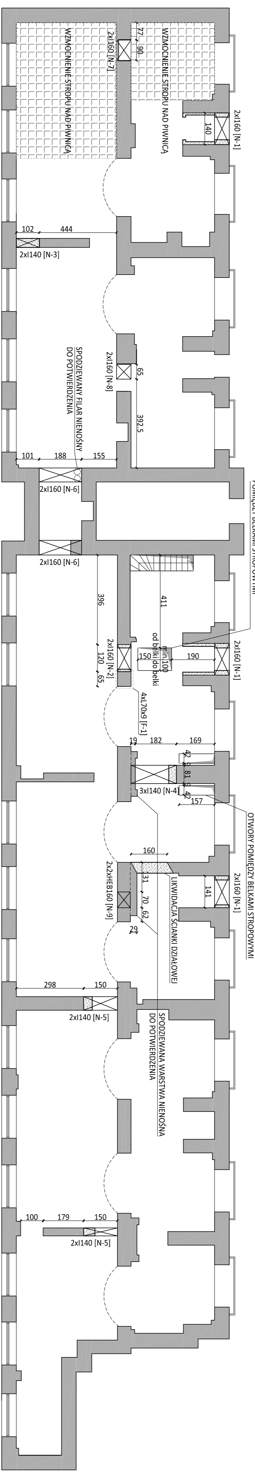
RZUT PARTERU SKALA 1:100
